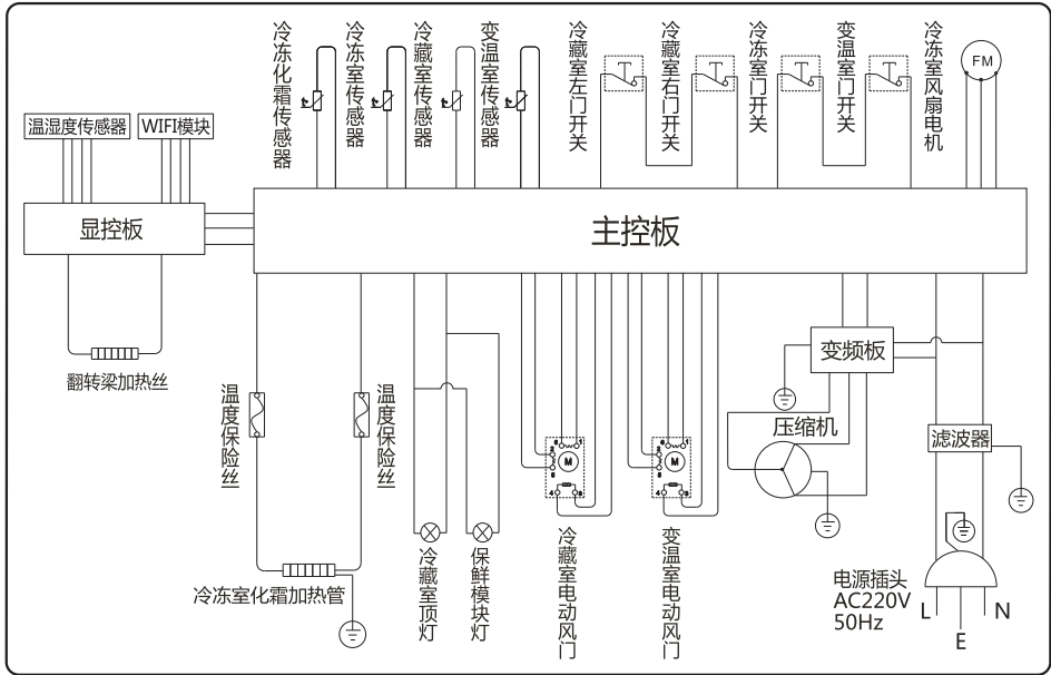
电路图 ( BCD-603WM01GBIWS )
